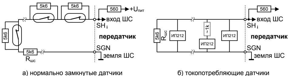
Рисунок 3 – Примеры монтажа пожарных шлейфов
