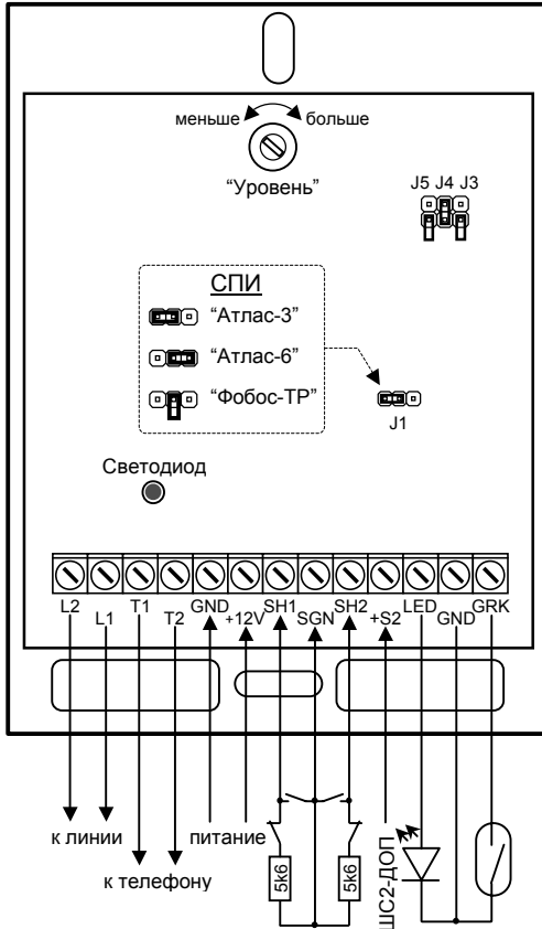
Рис. 4. Монтажная схема устройства исполнения “Риф Бастион-1-Ф”
