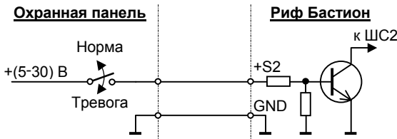
Рис. 3. Пример монтажа шлейфа ШС2-ДОП
