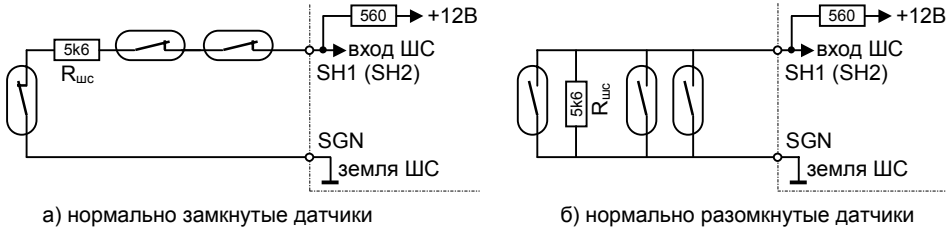
Рис. 2. Примеры монтажа шлейфов сигнализации
