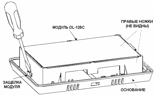
Рисунок 3. Отделение модуля от основания.
