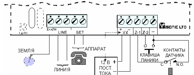
Рисунок 5. Электрические соединения DL-125C.
