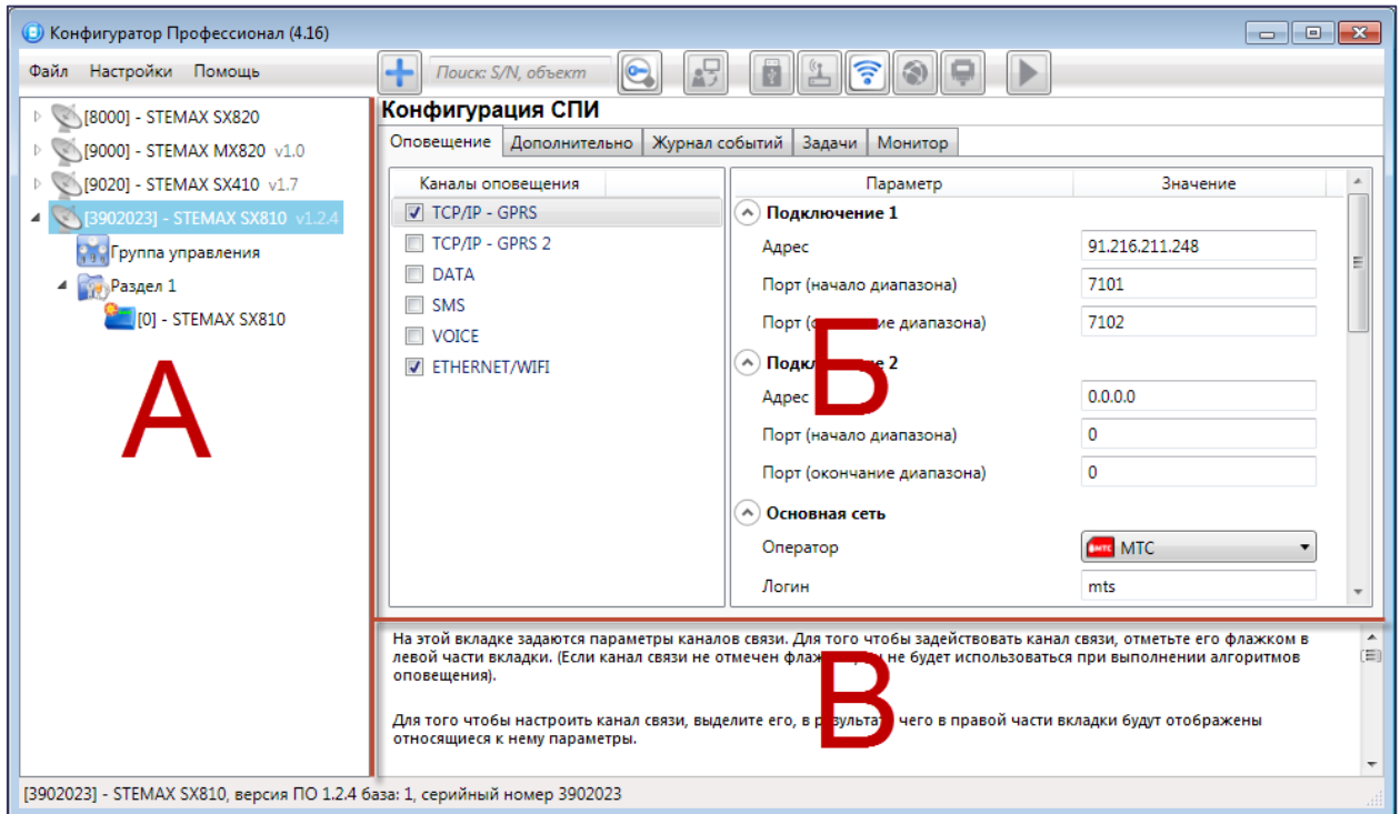
Рис. 5.1. Структура основного окна программы (А — дерево устройств, Б — область параметров, В — область подсказок)
