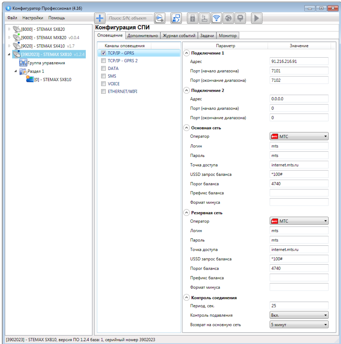
Рис. 5.6. Параметры канала TCP/IP - GPRS
