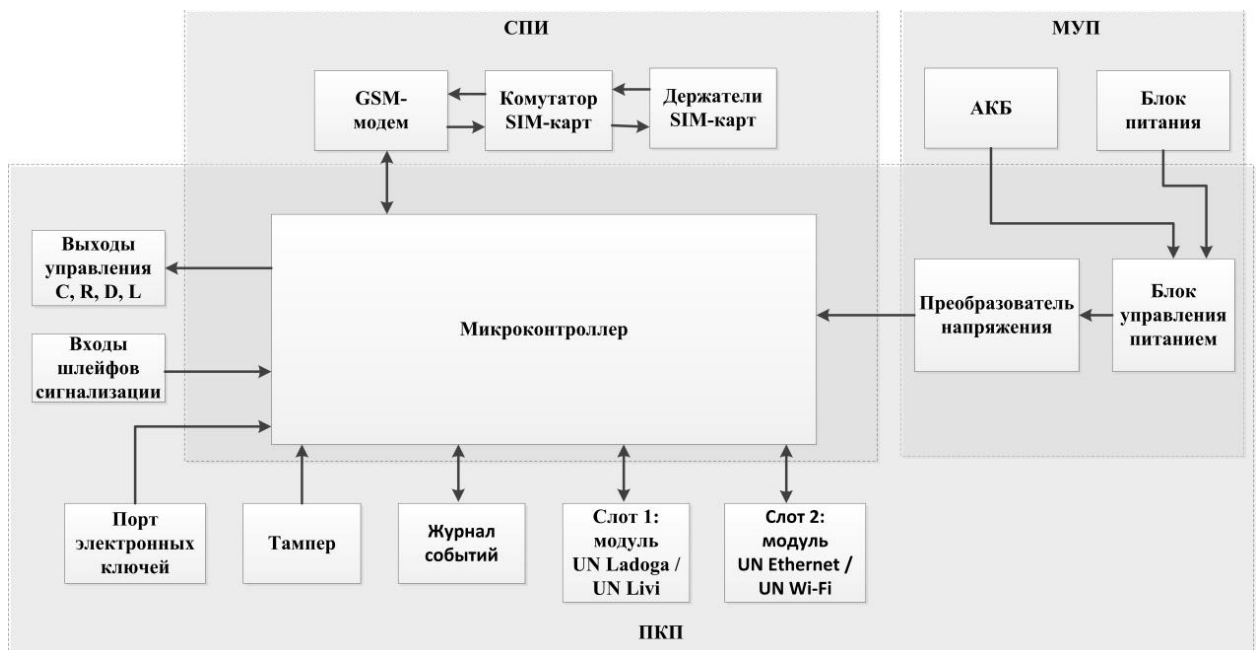
Рис. 3.1. Функциональная схема
