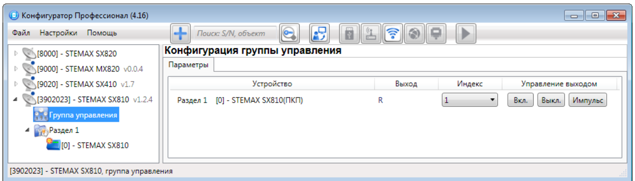
Рис. 5.43. Параметры и элементы дистанционного управления
