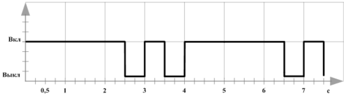
Рис. 14.3. Индикация режима На охране со шлейфом в состоянии Тревога и режима На охране с аварией
