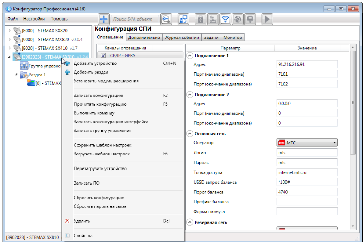
Рис. 6.1. Контекстное меню контроллера
