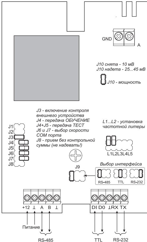
Рис. 2. Монтажная схема передатчика
