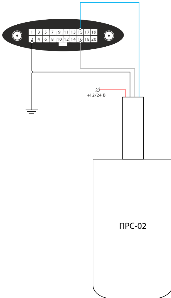
Рисунок 61. Схема подключения датчика контроля работы экскаватора
