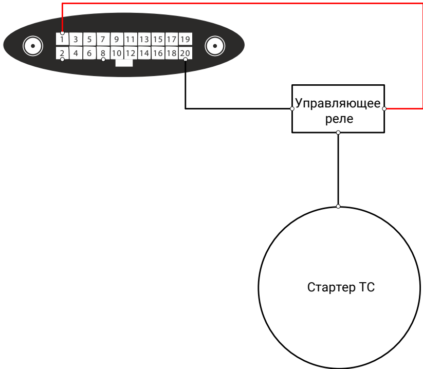
Рисунок 85. Схема подключения для блокировки стартера
