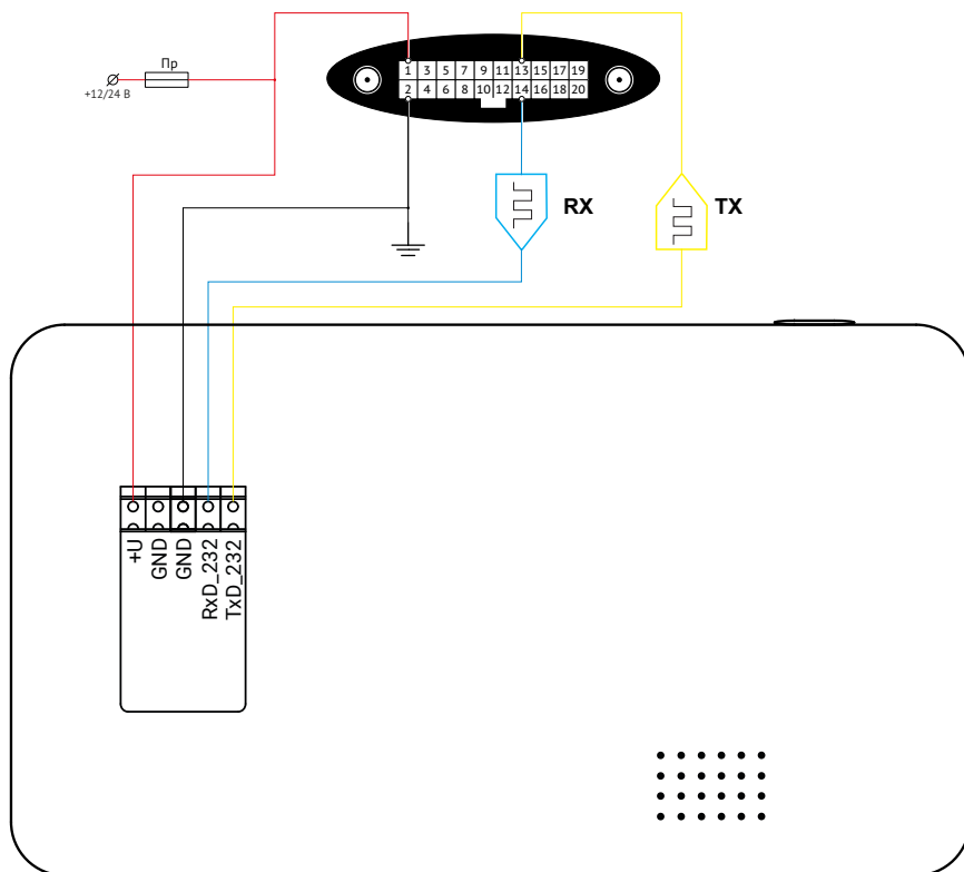
Рисунок 80. Схема подключения дисплея водителя
