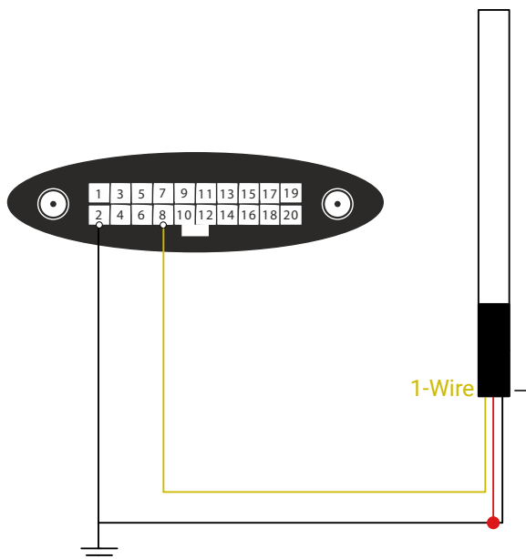
Рисунок 81. Схема подключения датчика температуры
