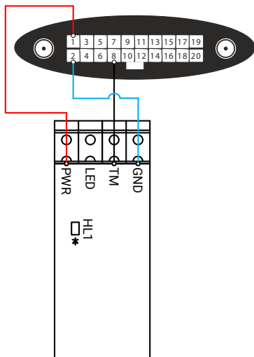
Рисунок 83. Схема подключения считывателя MIF
