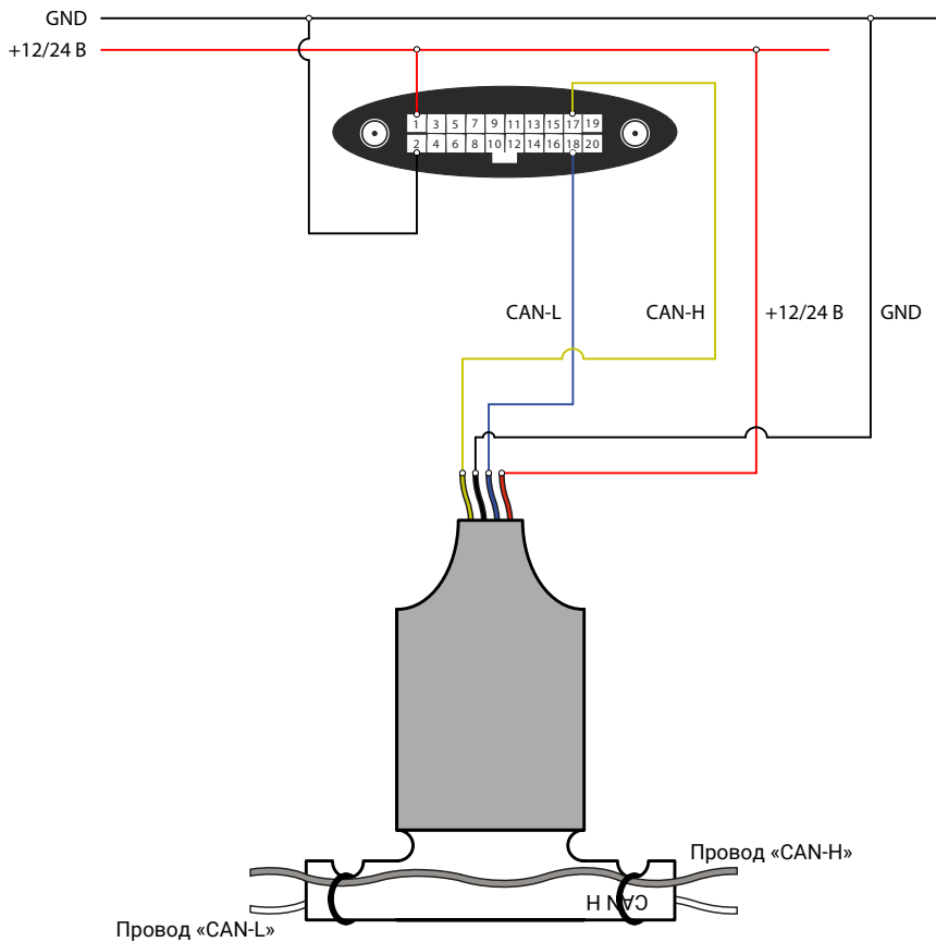
Рисунок 74. Подключение считывателя «CAN-IZOL-2»
