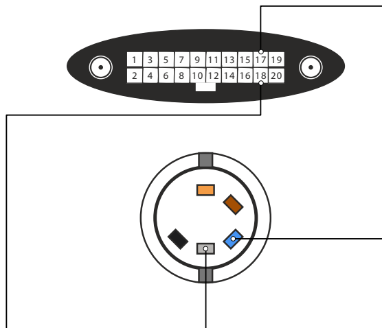
Рисунок 72. Подключение датчика DFM-250
