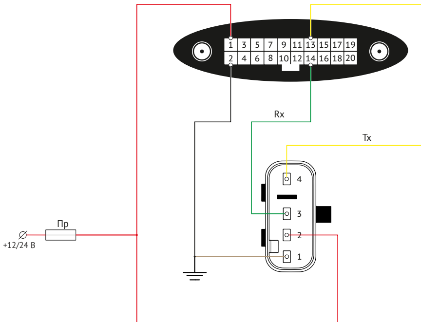
Рисунок 69. Схема подключения топливного датчика Стрела D232
