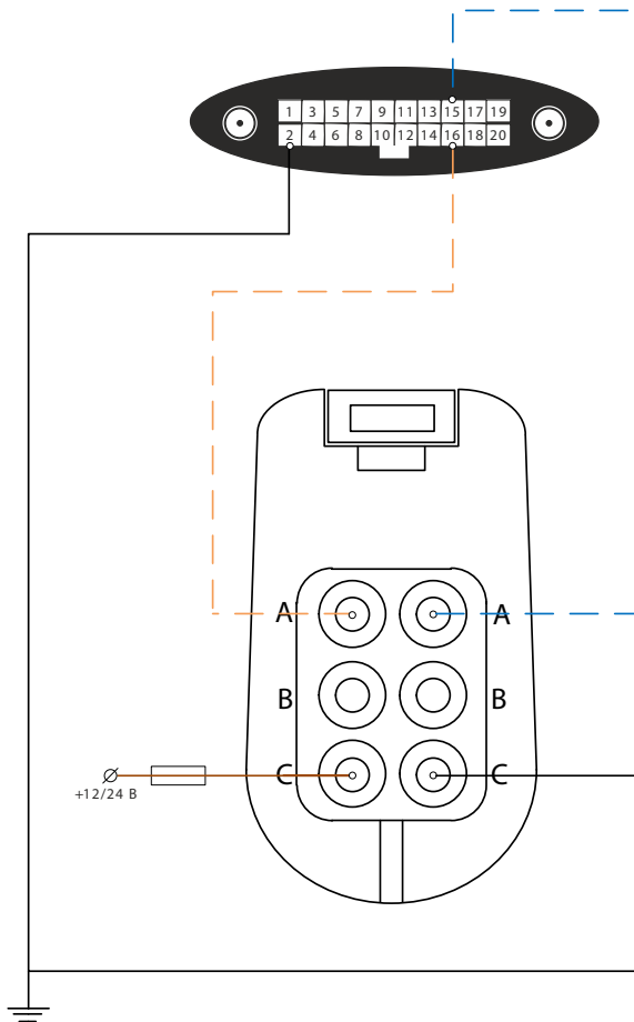
Рисунок 63. Схема подключения топливного датчика Omnicomm LLS-AF20160
