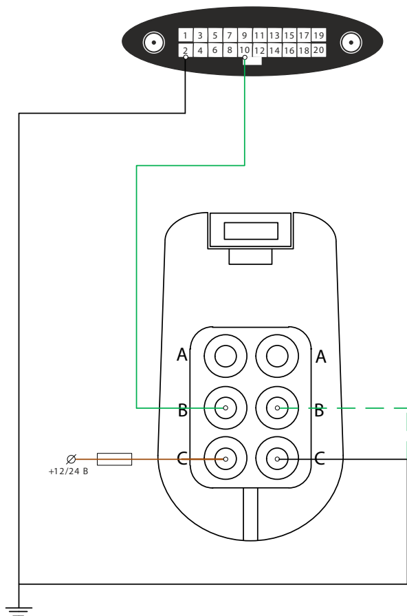
Рисунок 70. Схема подключения частотно-аналогового датчика
