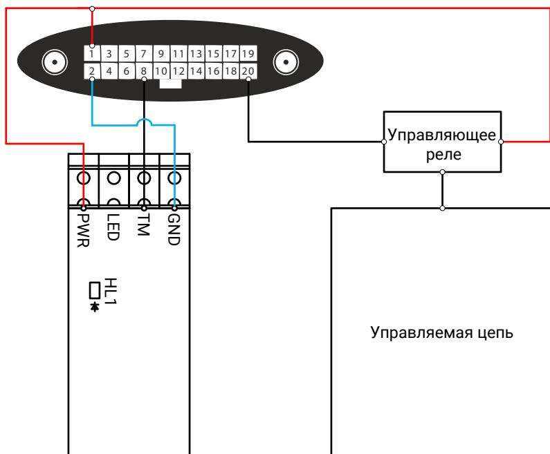
Рисунок 84. Схема подключения блокируемой цепи
