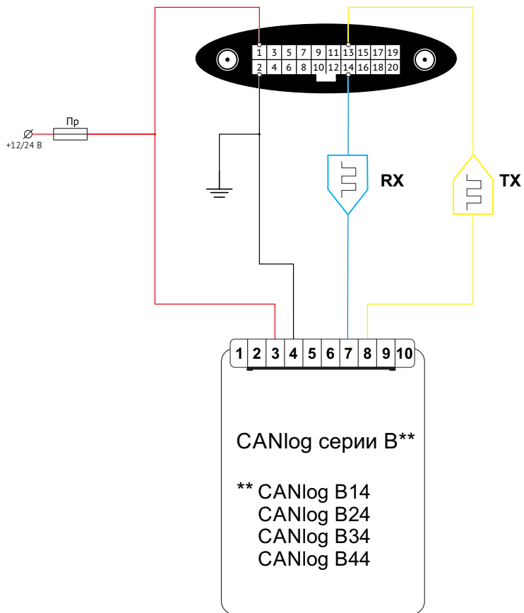
Рисунок 75. Подключение считывателя «CAN-LOG»
