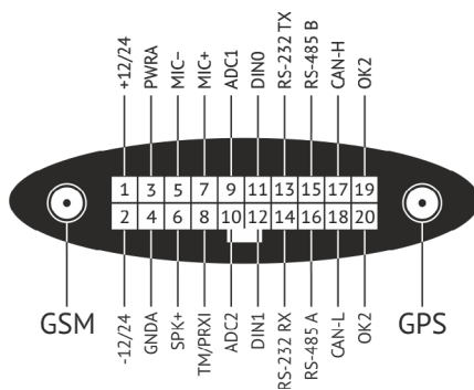
Рисунок 58. 20-контактный разъем трекера
