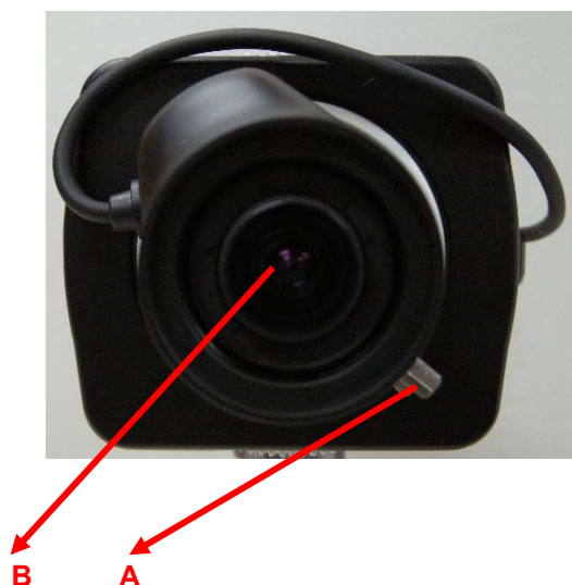
Рисунок 2. Вид спереди MDC-i4270C, MDC-i4270CTD
