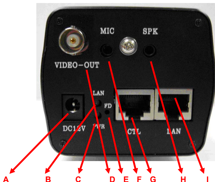
Рисунок 3. Вид сзади MDC-i4270C, MDC-i4270CTD
