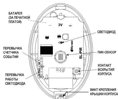
Рисунок 2. Вид изнутри
