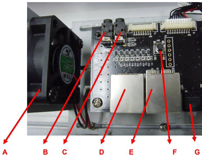
Рисунок 3. Внутренние части MDC-i6261VTD-66H
