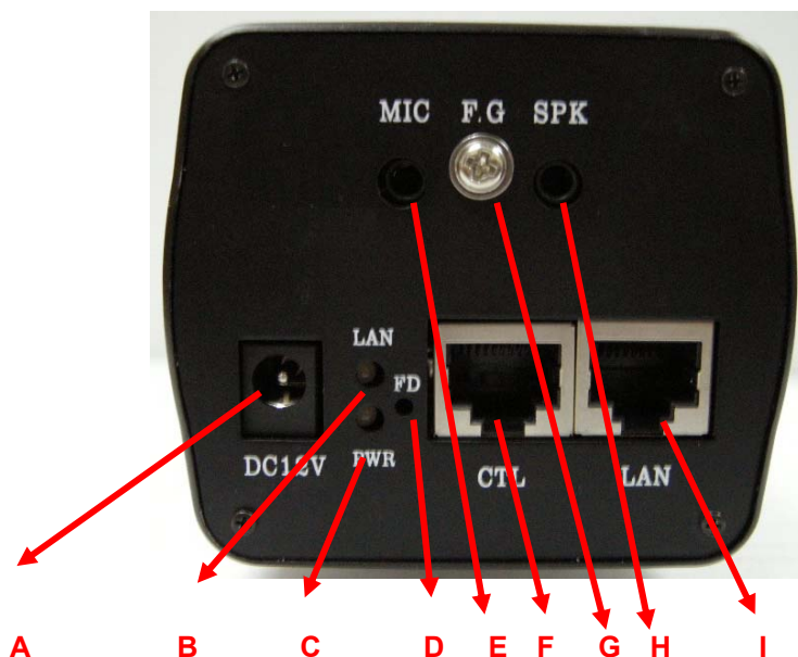
Рисунок 3. Вид сзади MDC-i4250C, MDC-i4250CTD
