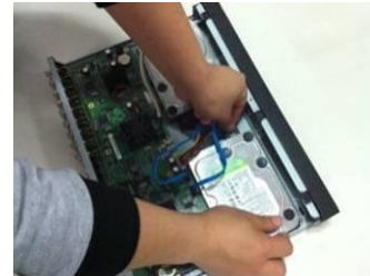
Падключыце SATA кабель і кабель харчаванн на ніжняй і задняй частцы корпуса і зачыніце корпус верхняй вешкам.
